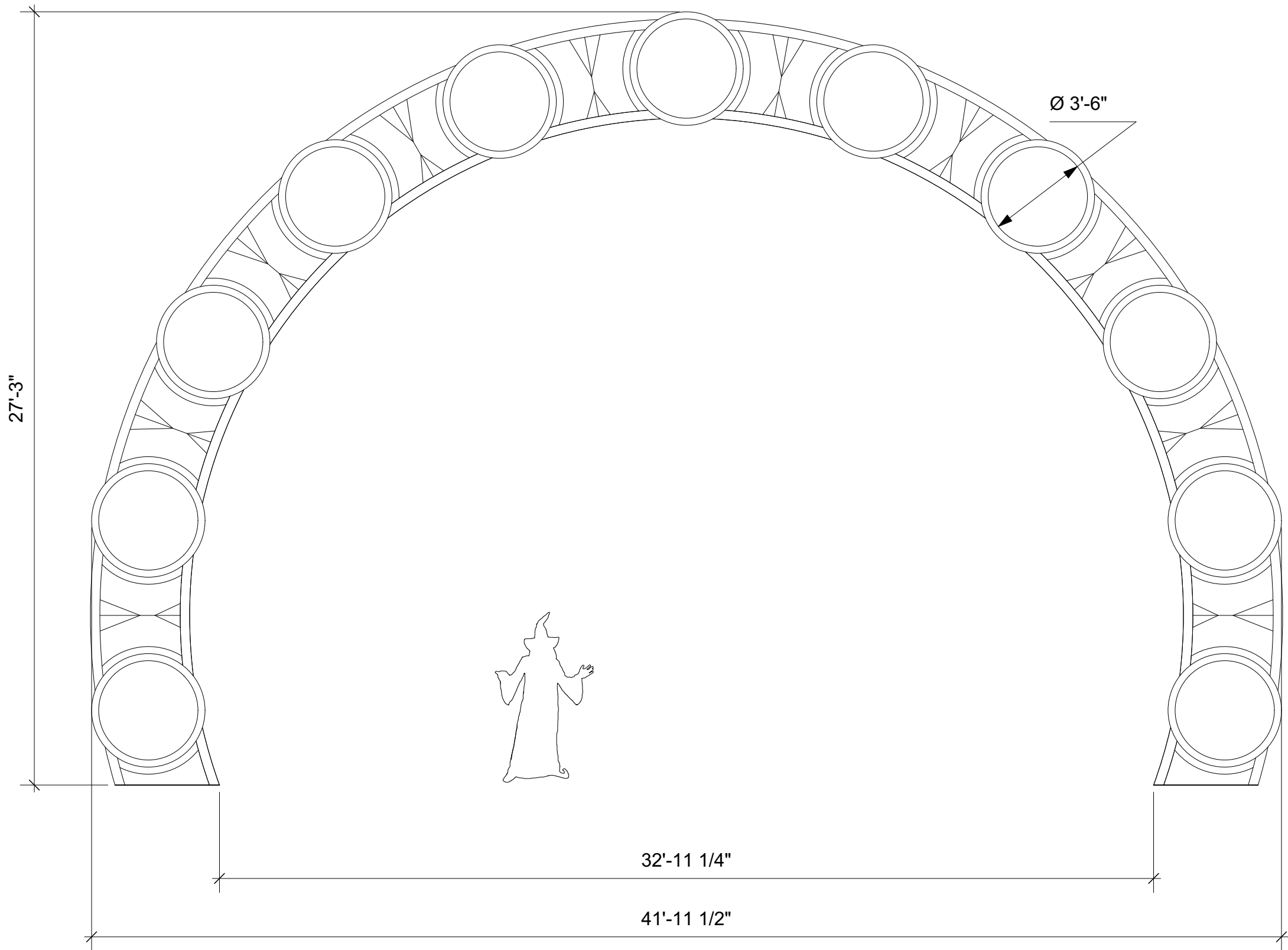
17 Portal Scale: 1/4" = 1'-0"
